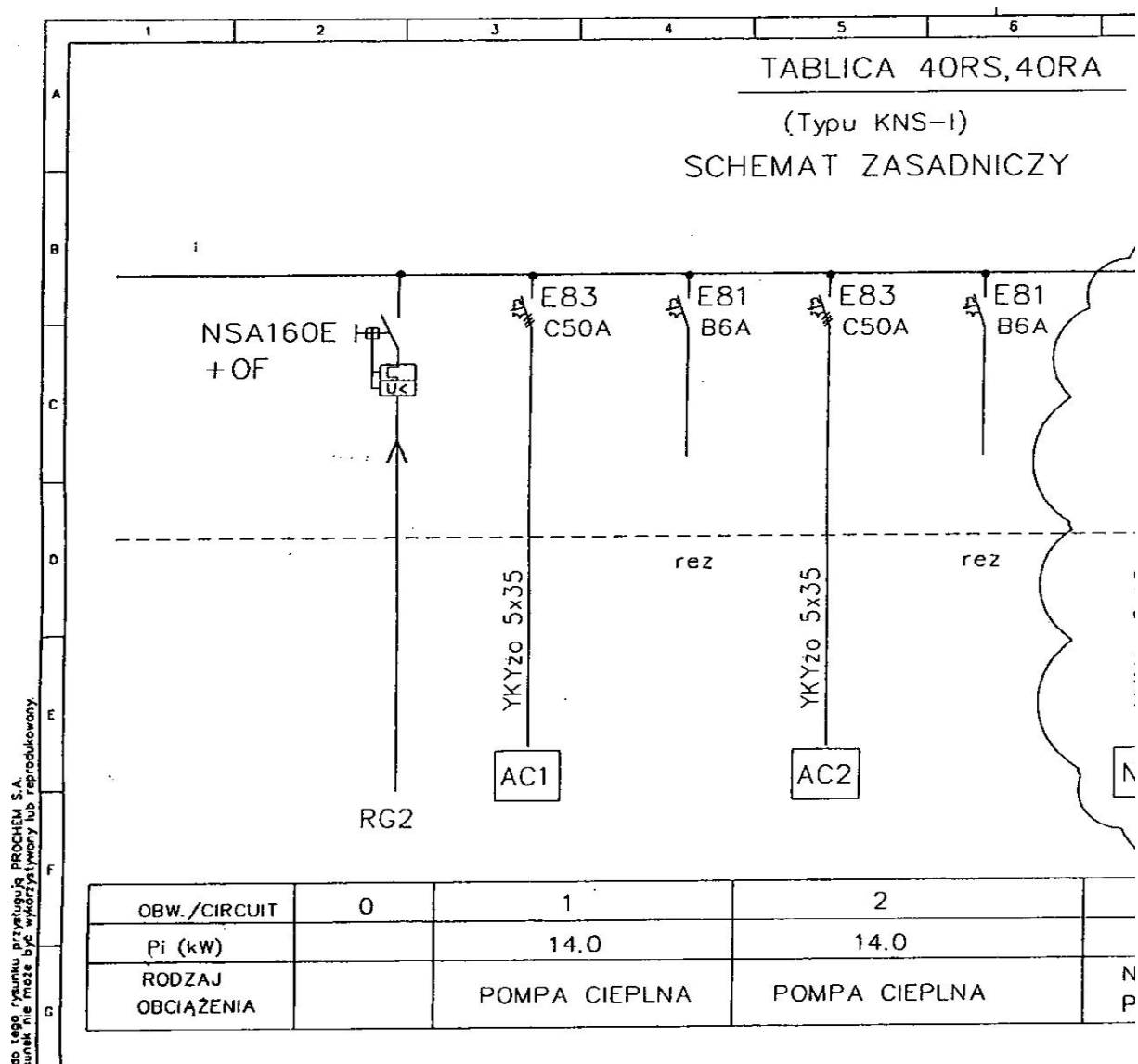
Rys. nr 4 Zasilanie pomp ciepła TWR
