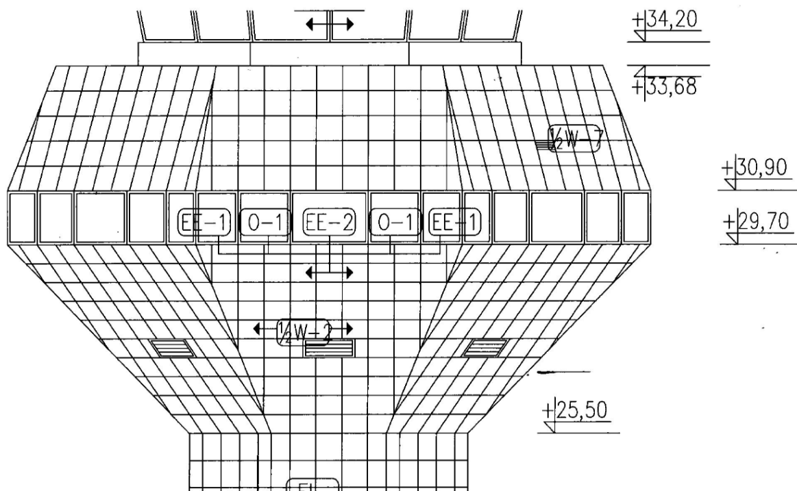
Rys. nr 5 Rzut wieży TWR
