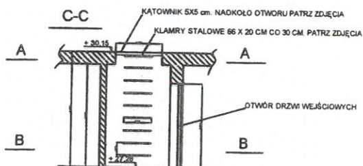
SZACHT DOJŚCIA TECHNICZNEGO PRZEKRÓJ C-C
