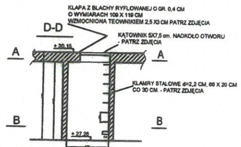
SZACHT DOJŚCIA TECHNICZNEGO PRZEKRÓJ D-D
