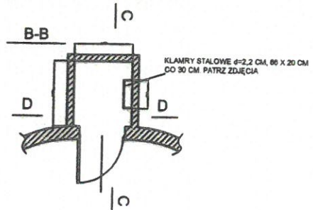
SZACHT DOJŚCIA TECHNICZNEGO - CZĘŚĆ DOLNA PRZEKRÓJ B-B
