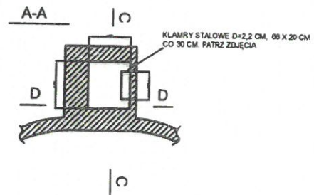
SZACHT DOJŚCIA TECHNICZNEGO - CZĘŚĆ GÓRNA PRZEKRÓJ A-A
