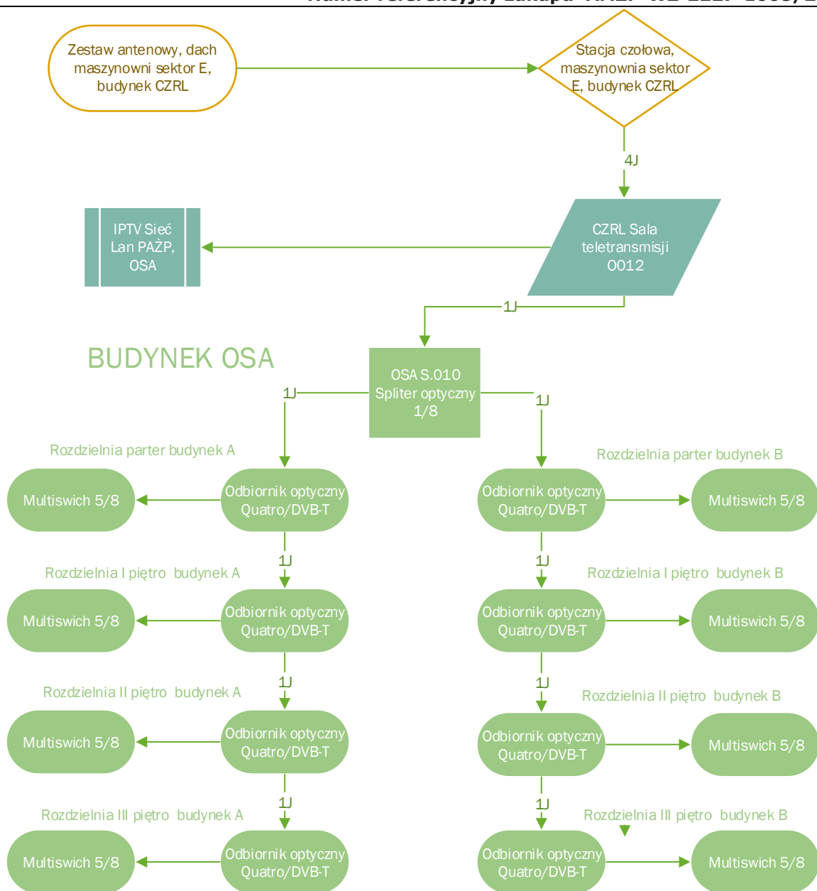
Rys 1. Schemat planowanej instalacji antenowej w budynku OSA PAŹP.
