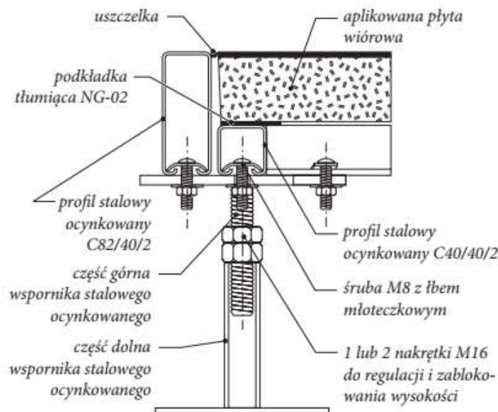
Schemat konstrukcji nośnej podłogi podniesionej
